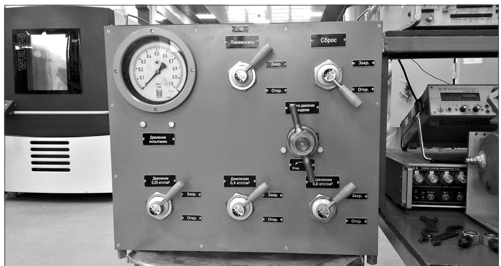
Стенд пневматический С185.
